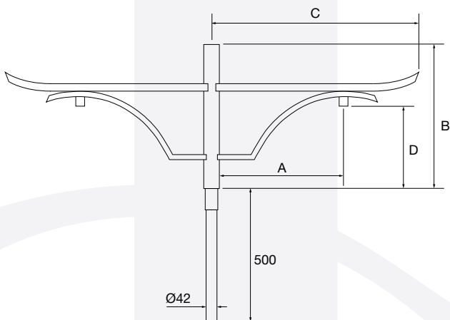
CHERBOURG 2 FEUX / 2 LIGHTS
